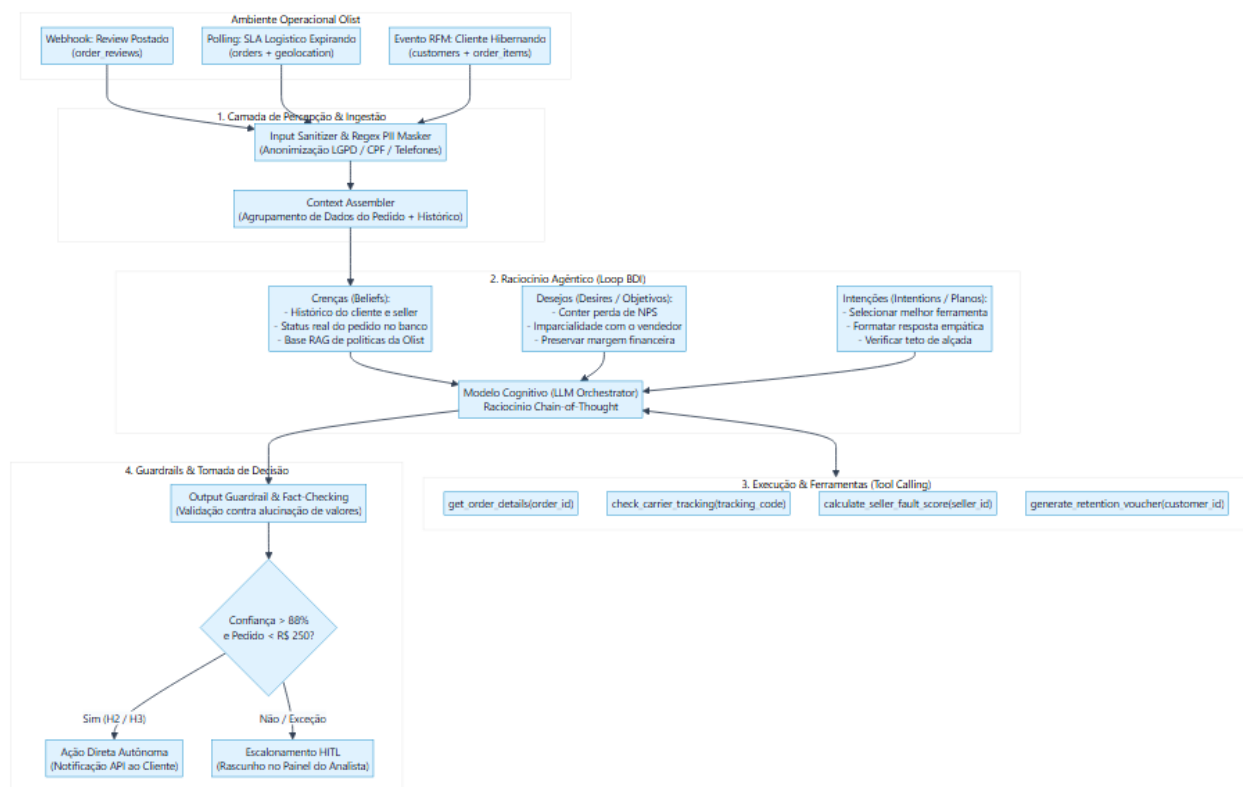
Figura 10 — Arquitetura Cognitiva do Loop BDI (Percepção - Raciocínio - Ação com Tool Calling e Guardrails)
